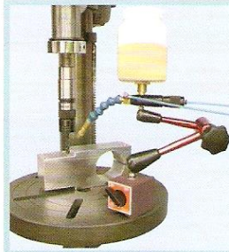
眼鏡蛇噴油器 Cobra Lubricator System TM 800031
